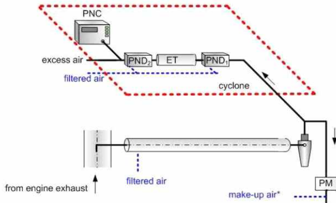
그림 1. 최적 입자개수 측정장치(부분유량 채취시스템)
